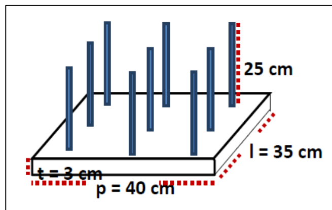
Gambar 2. Sketsa kerangka dan spesifikasi ukuran bioreeftek
