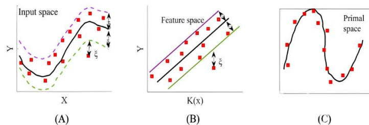
Gambar 1 Ilustrasi Konsep SVR
