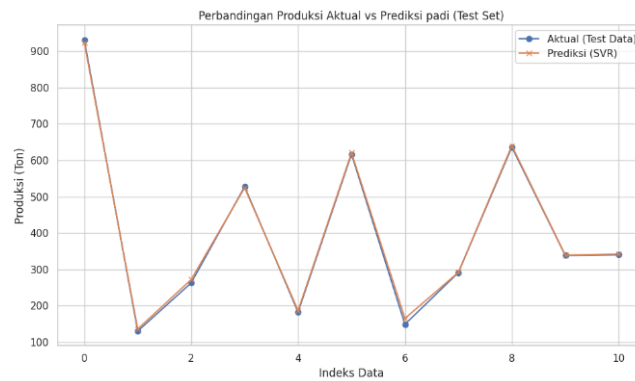
Gambar 3. Visualisasi Prediksi Padi
