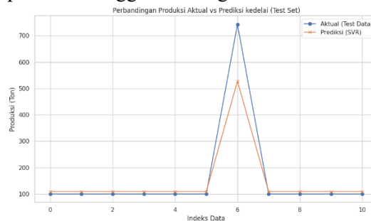
Gambar 5. Visualisasi Prediksi Kedelai.
