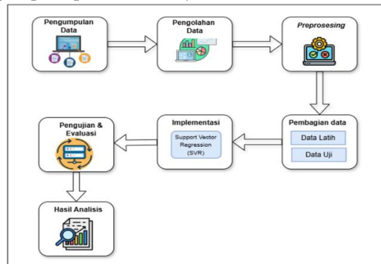
Gambar 2. Tahapan penelitian
