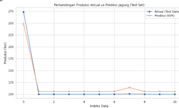
Gambar 4. Visualisasi Prediksi Jagung
