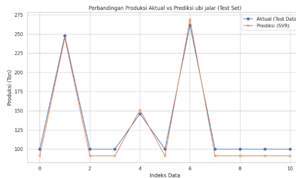
Gambar 9. Visualisasi Prediksi Ubi Jalar.
