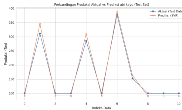
Gambar 8. Visualisasi Prediksi Ubi Kayu.
