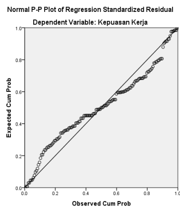
Gambar 1. Uji Normalitas
