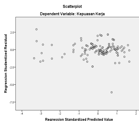
Gambar 2. Uji Heteroskedastisitas
