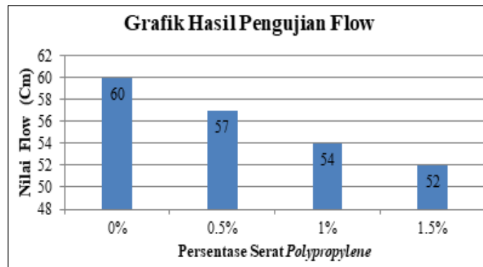
Gambar 1. Grafik Hasil Pengujian Flow
